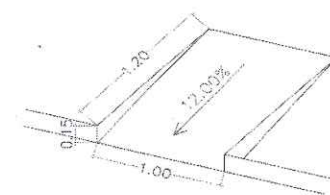
Detalle de rampa tipo
