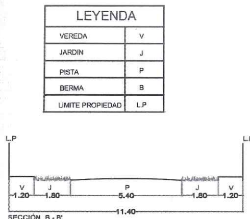
SECCIÓN B - B'
