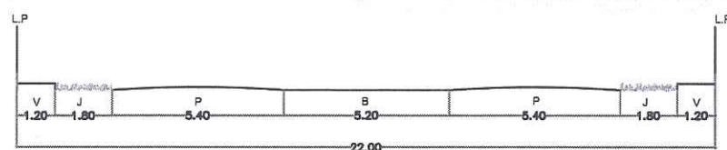
SECCIÓN A1 - A1'
