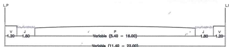
SECCIÓN A - A'
