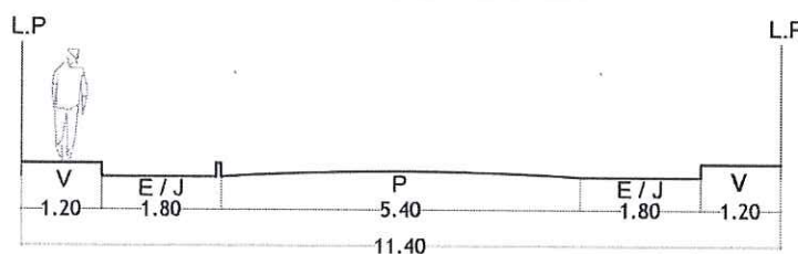
SECCIÓN 35 - 35
