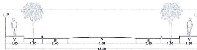
SECCIÓN 66 - 66
