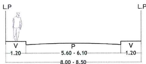
SECCIÓN G2 - G2
