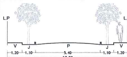
SECCIÓN 67 - 67
