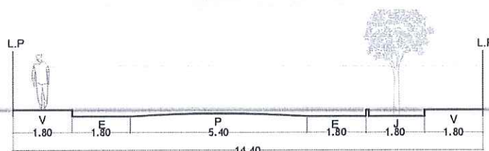
SECCIÓN 94 - 94
