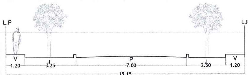
SECCIÓN G3 - G3
