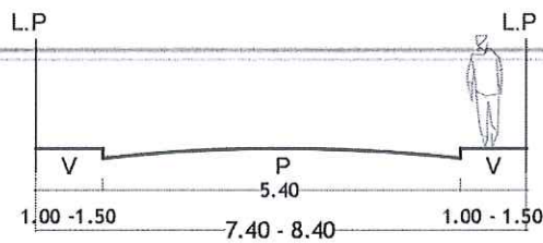
SECCIÓN 56 - 56
