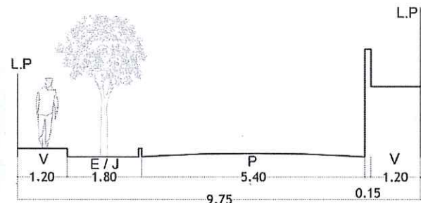
SECCIÓN 65 - 65
