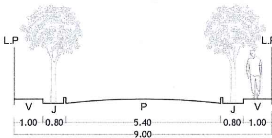
SECCIÓN 64 - 64
