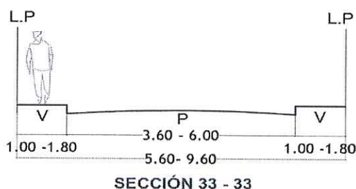
SECCIÓN 33 - 33
