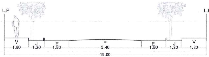
SECCIÓN 48 - 48
