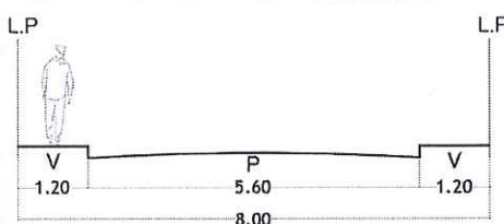
SECCIÓN G1 - G1
