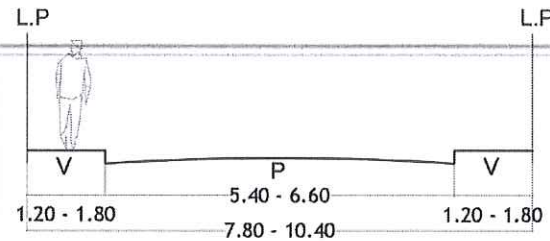
SECCIÓN 60 - 60
